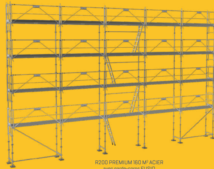
R200 PREMIUM 160 M 2 ACIER avec garde-corps FUSIO
